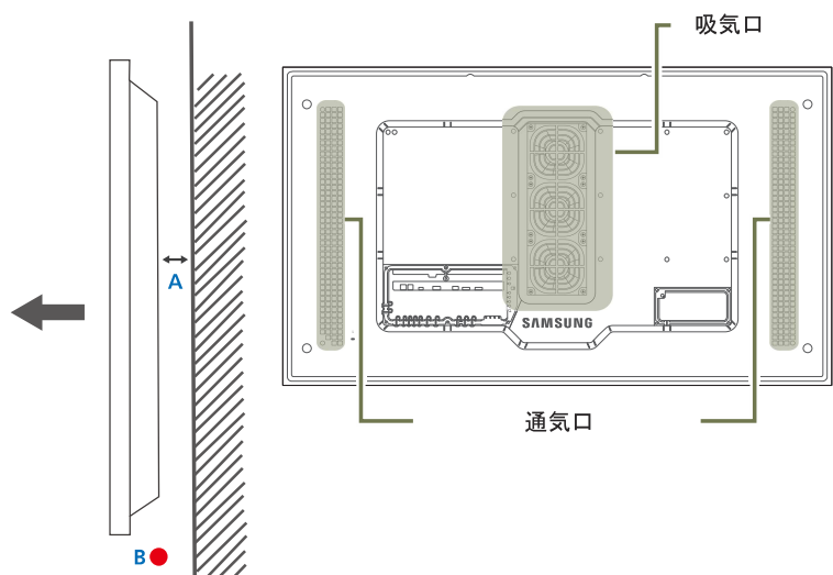
図 1.1 側面図
